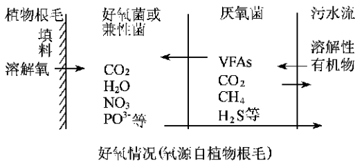
图2 植物根毛释放氧气作用下湿地中的物质传递及变化过程
